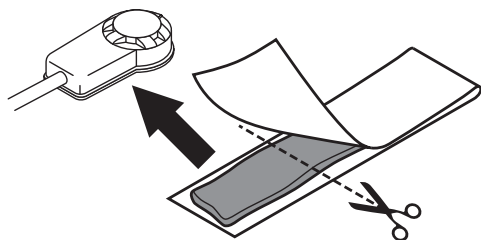
Abbildung 5: Klebemasse auf die Unterseite des Pickups drücken
