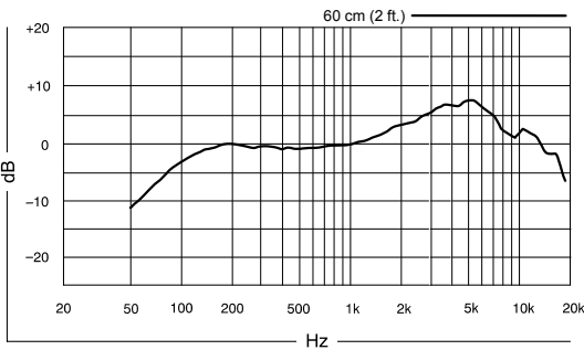
Типичная частотная характеристика
