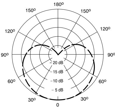
Patrón polar de captación típico
