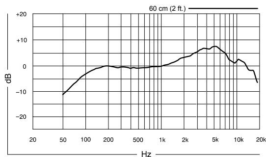
Typische frequentiekenarakteristiek
