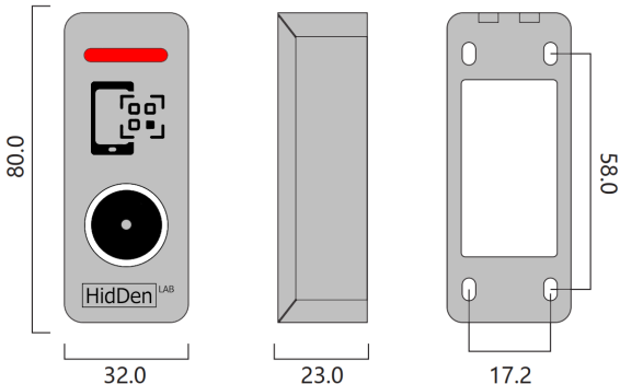
Рис.3 QR-X-5. Габариты.
