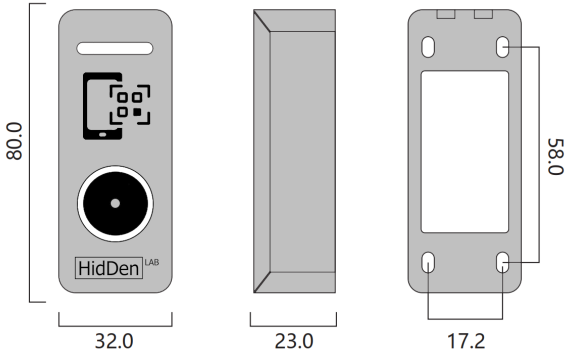
Рис.2 QR-X-4. Габариты.
