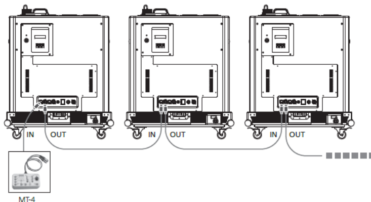
Подключение других генераторов тяжелого дыма AQUAFOG 2500 или AQUAFOG 3600
