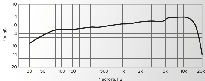
Амплитудно-частотная характеристика
